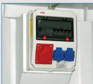
salvavita con prese elettriche integrate
